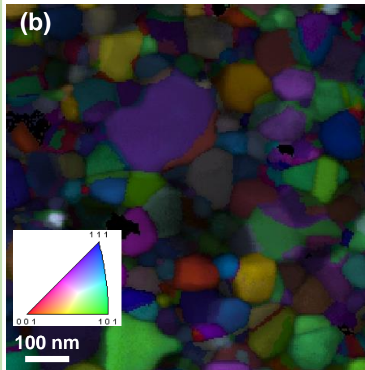
IPF
