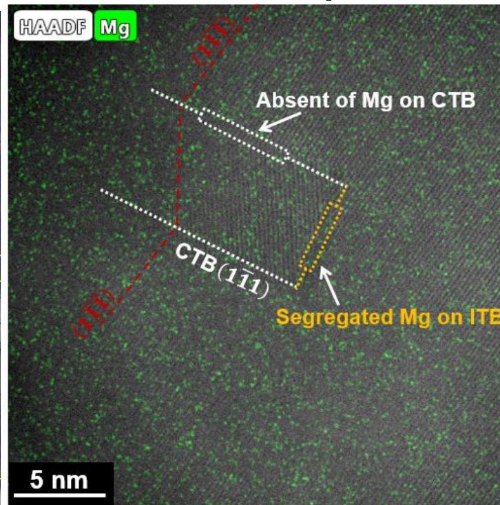
EDS Map
