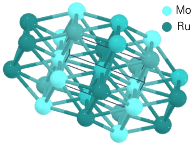
Fig. 1. Mo-Ru Alloy
