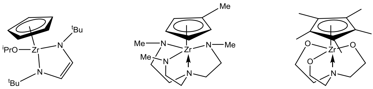
Zr(Cp)( t BuDAD)(O i Pr), Zr(MeCp)(TMEA) and Zr(Me 5 Cp)(TEA) precursors
